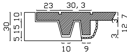
DETALLE B (tapa)
