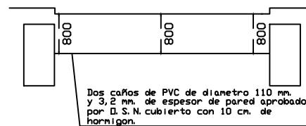
DETALLE CRUCE DE CALLE
