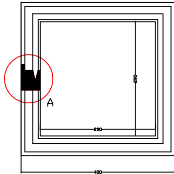
DETALLE A (marco)
