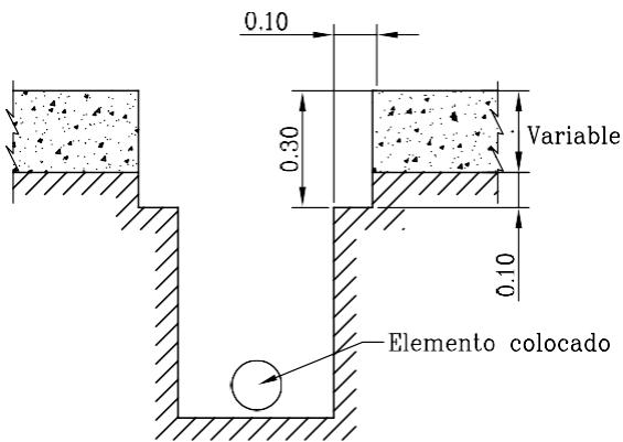
(b) CORTE
