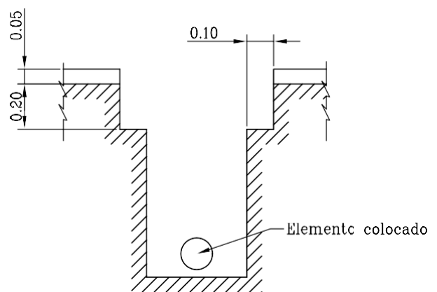
(b) CORTE
