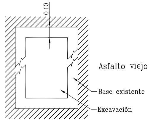
(a) PLANTA
