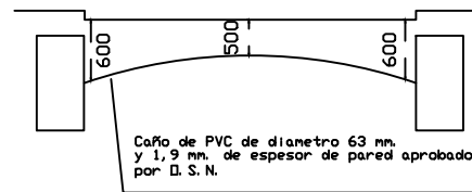
DETALLE ENTRE CAJAS
