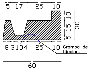
DETALLE A (marco)
