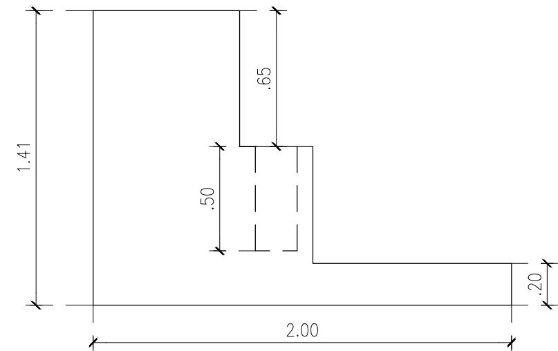
VISTA LATERAL
